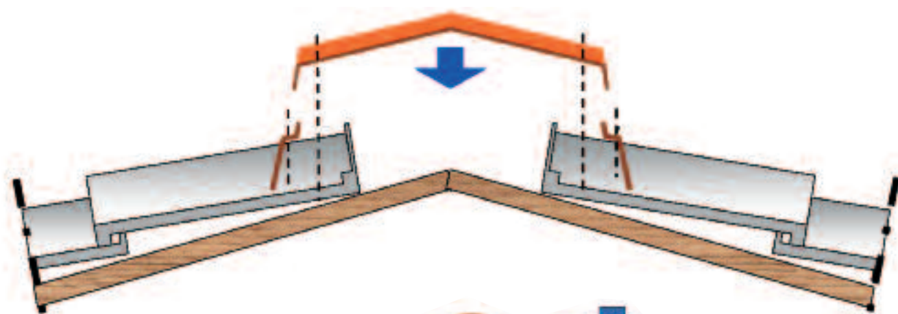
Art. LISS.PR-C Listello chiudi coppi principale per colmo per SENESE ml utili: 0,93
